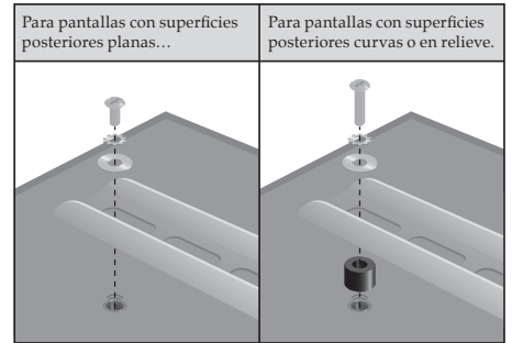
Fig. 3 – Utilice un perno más largo y un separador para pantallas con superficies posteriores curvas o en relieve. No utilice la Arandela M6 (O) si está usando Pernos M8 (J o K).
